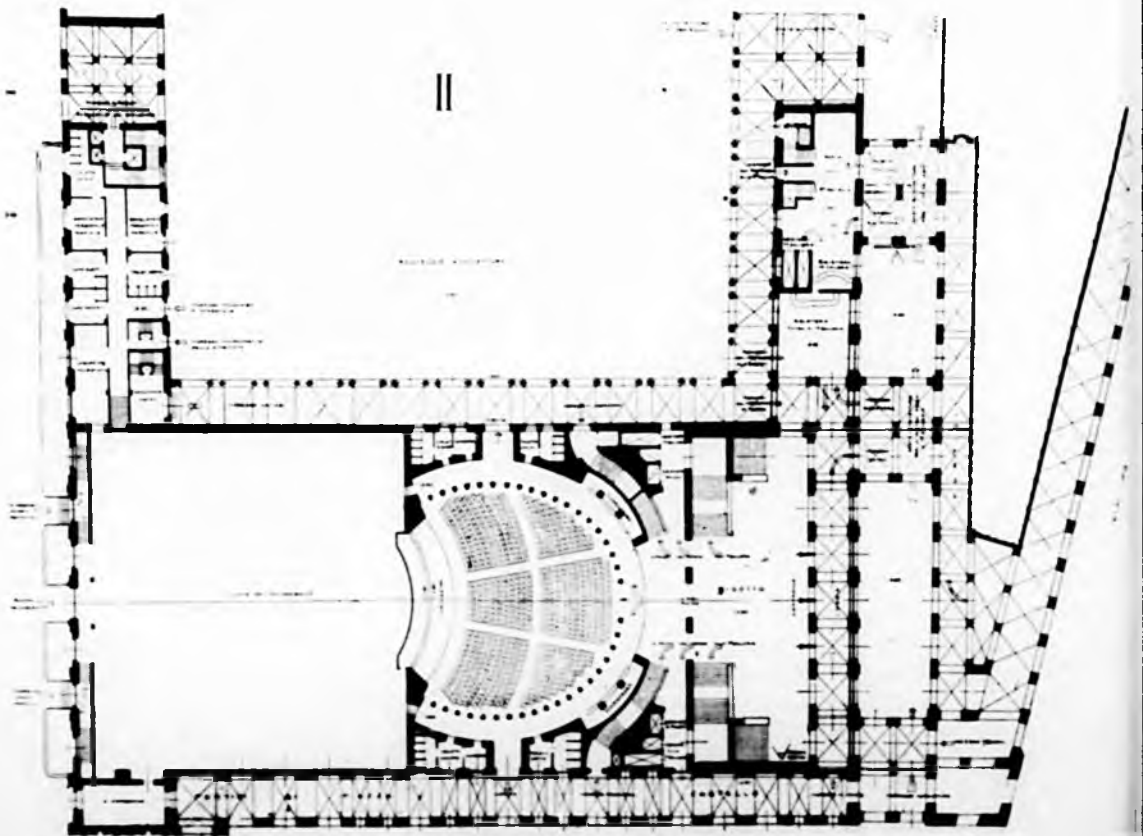
Pianta a piano terra del Progetto (B)
