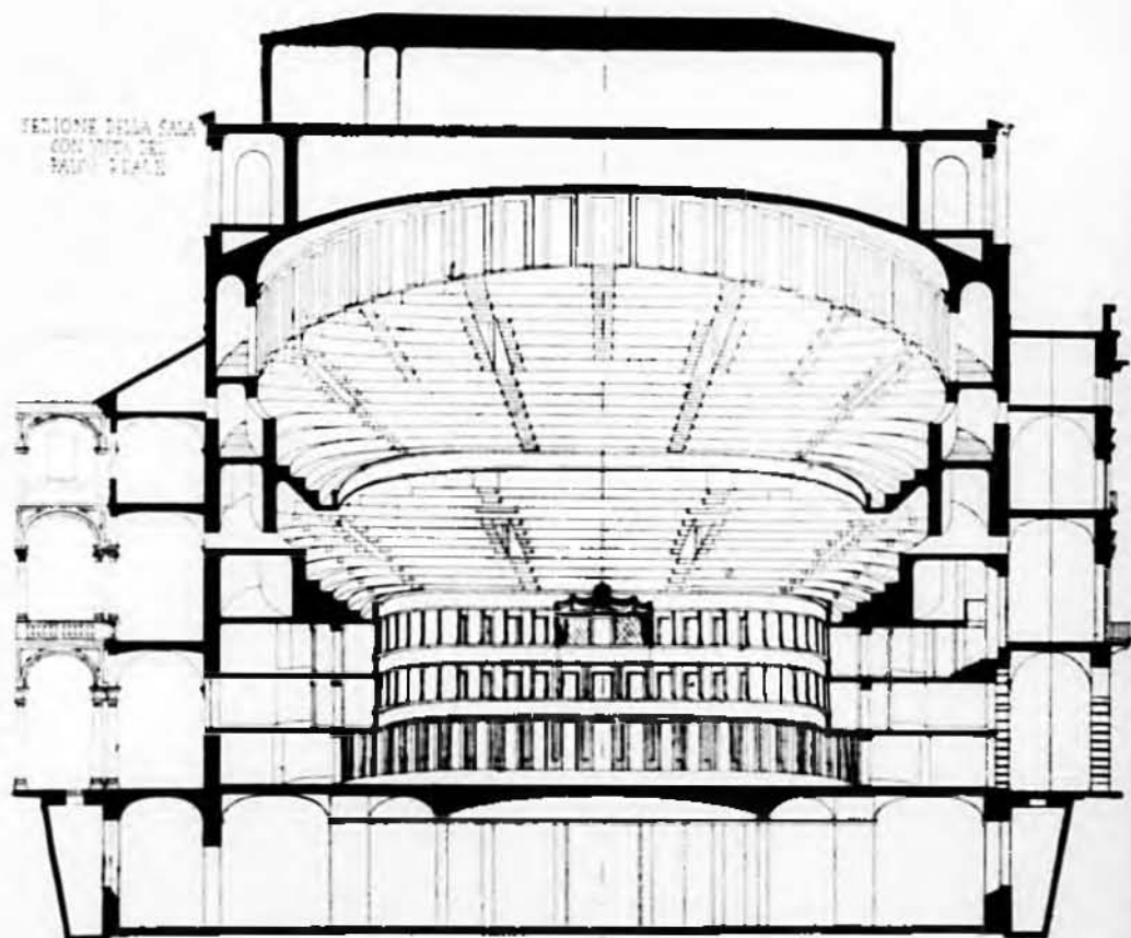
Sezione trasversale
