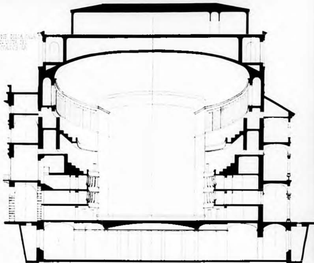
Sezione trasversale
