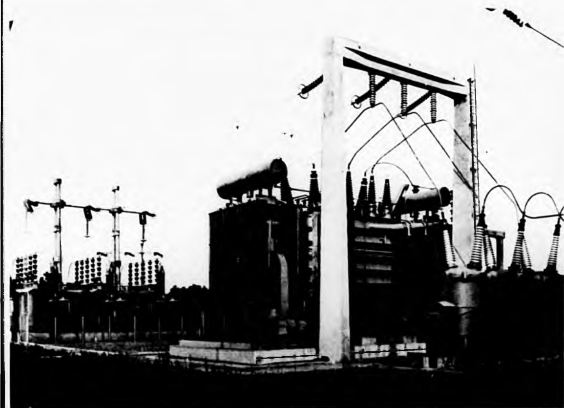
Fig. 6. Veduta della Sottostazione di Turbigo - trasformazione da 220.000 Volt a 135.000 Volt
